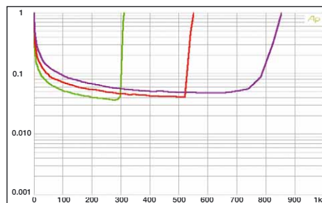
Satte Leistung an allen Lasten bis 1 Ohm. Der Klirr hält sich angenehm in Grenzen
