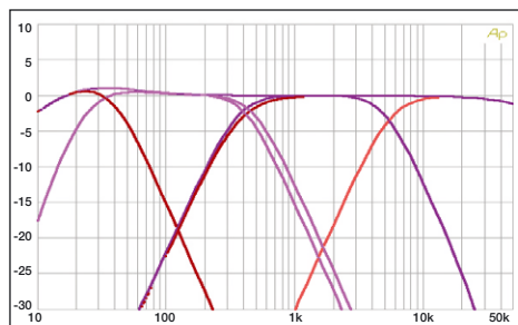
Durch die x10- und x15-Schalter lässt sich der Wirkungsbereich der Frequenzweichen von 22 Hz bis 5,5 kHz ausdehnen
