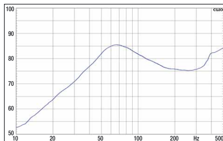
Der HX zeigt in geschlossenen 30 Litern einen flacheren Bassabfall als in Bassreflex, -3 dB bei knapp 50 Hz sind keine Tiefbassorgien
